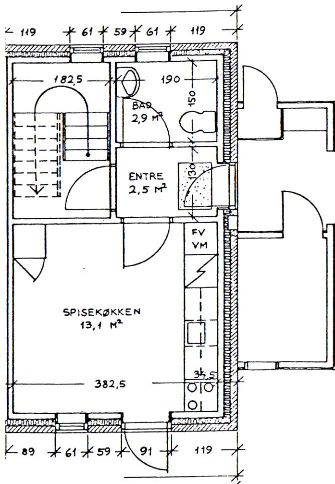
Plan af stueetage
